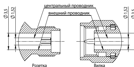
Соединители 3,5 мм и IX, розетка и вилка
