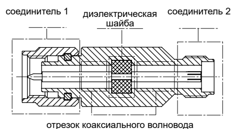
Устройство перехода
