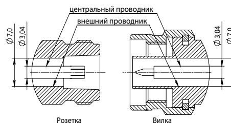
Соединители N и III, розетка и вилка
